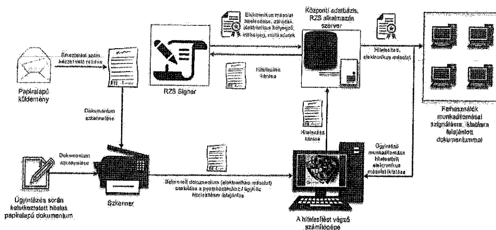
I. ábra: Papíralapú dokumentumról hiteles elektronikus másolat készítésének rendszerszintű feldolgozási folyamata
