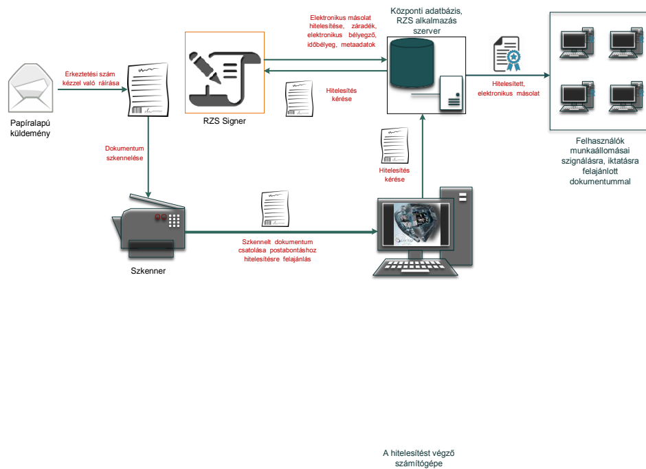
1. ábra: Papíralapú iratról hiteles elektronikus másolat készítésének rendszerszintű feldolgozási folyamata
