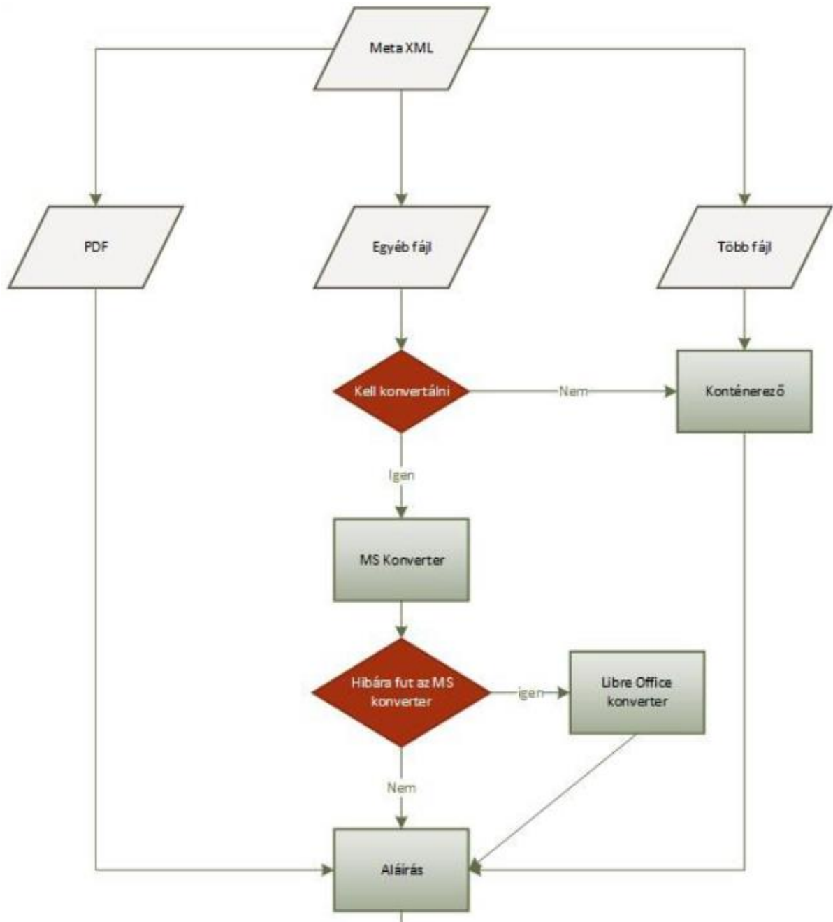
3. ábra RZS Signer rendszerszintű működése
