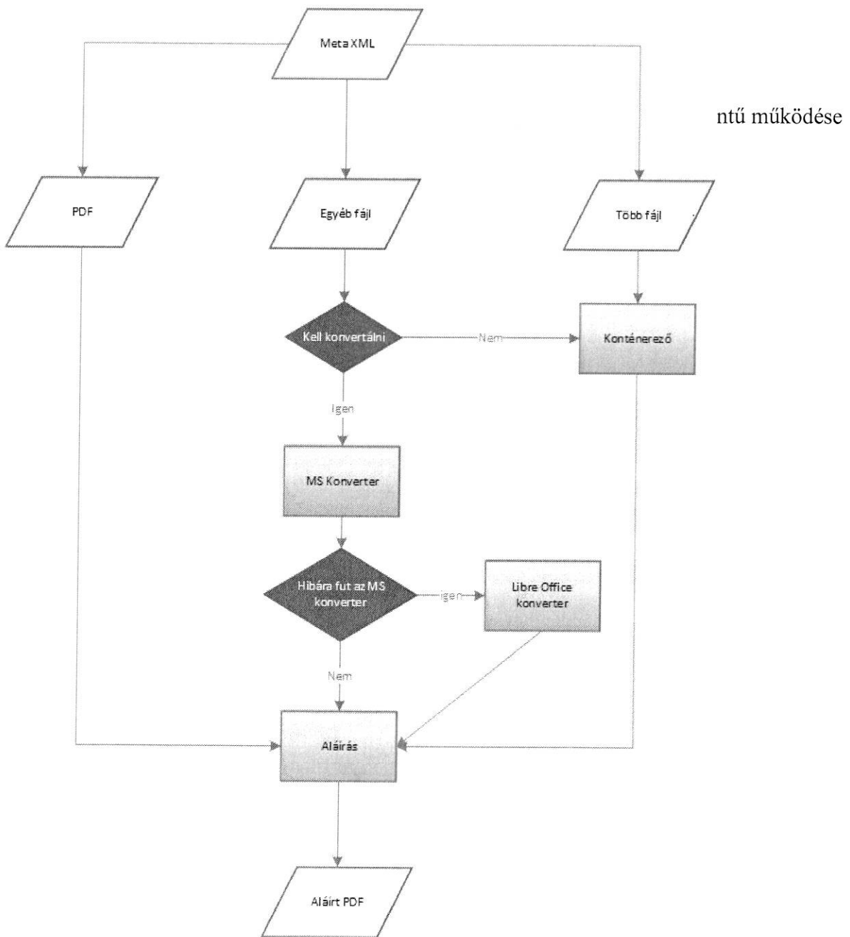
ábra: Az RZS Signer hitelesítés funkció rendszerszintű működése
